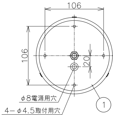
取付部寸法
