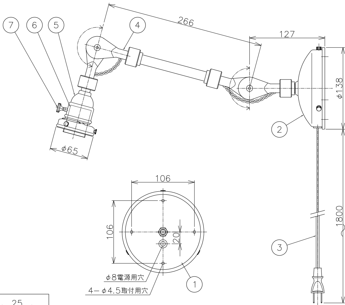
取付部寸法
