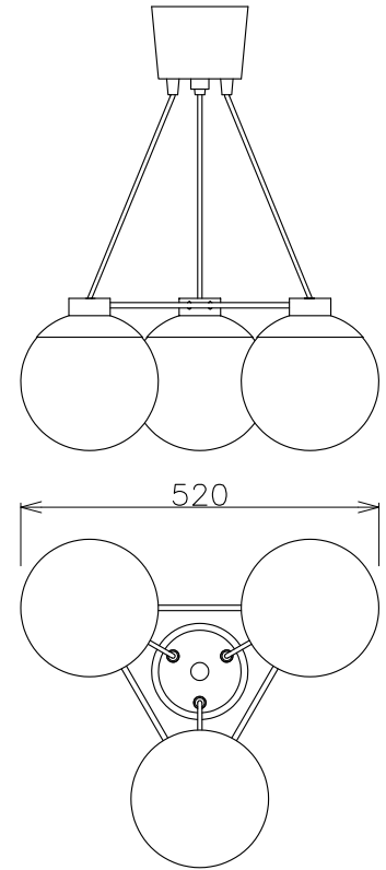
別取付例 尺度1/12 トライアングル(三角形)
