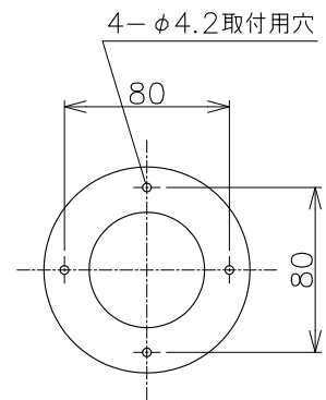
取付部寸法
